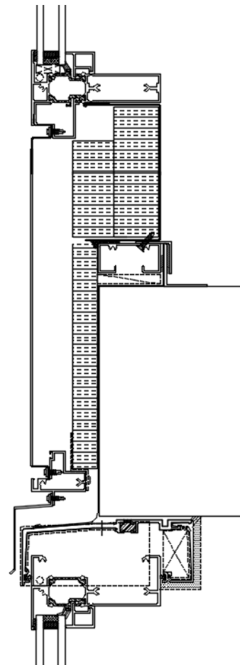
EXTERIOR: TOP HAT PANEL INTERIOR: ALUMINUM BACK PAN
