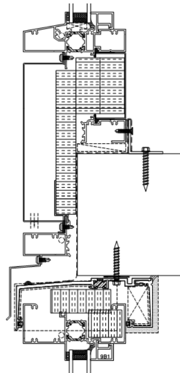
EXTERIOR: TOP HAT PANEL INTERIOR: ALUMINUM BACK PAN
